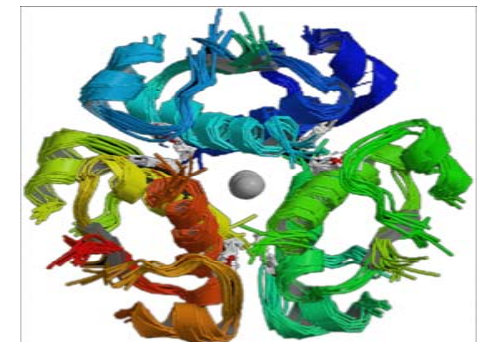
INSULIN-MOLEKÜLE
